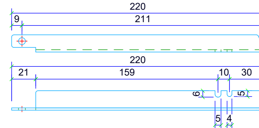
Füsse / 2 Stück wie gezeichnet
