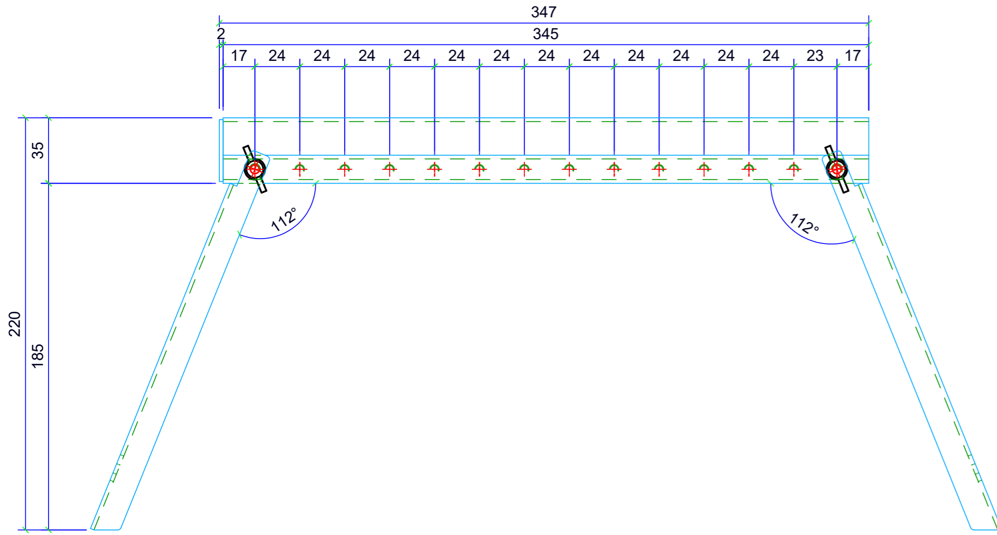
Ansicht Grill
