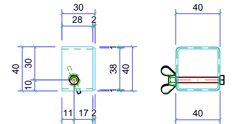
Abschluss-Deckel
