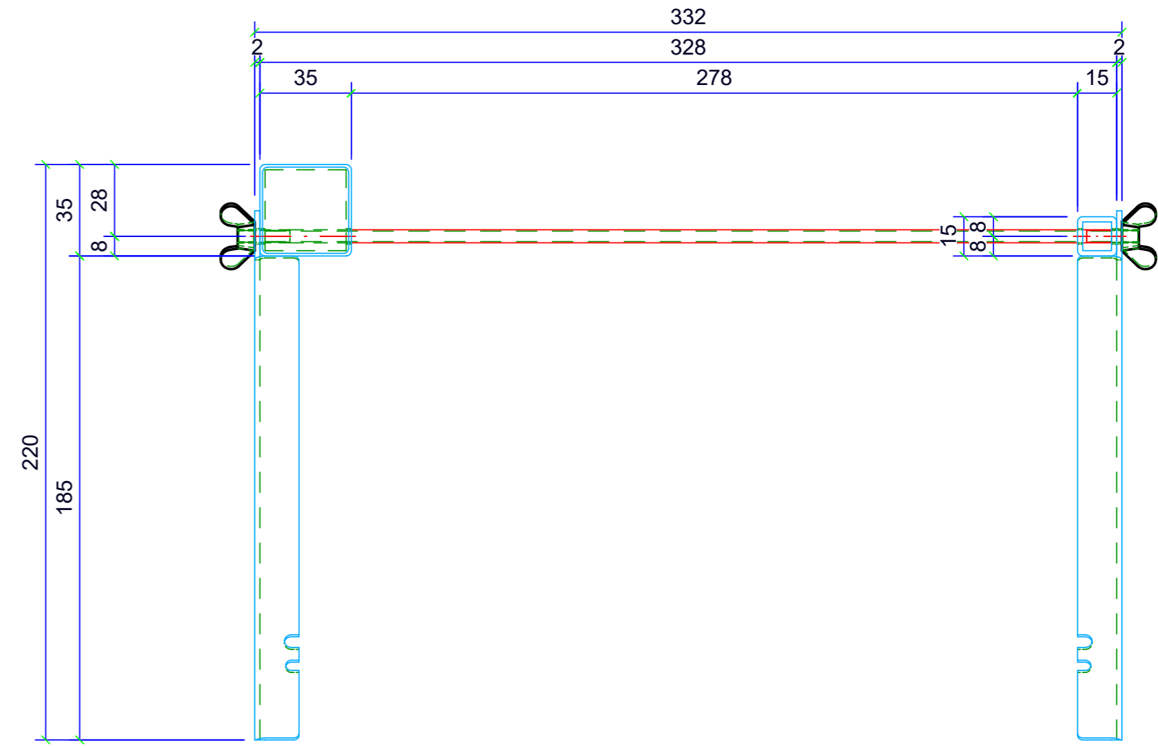
Seitenriss Grill
