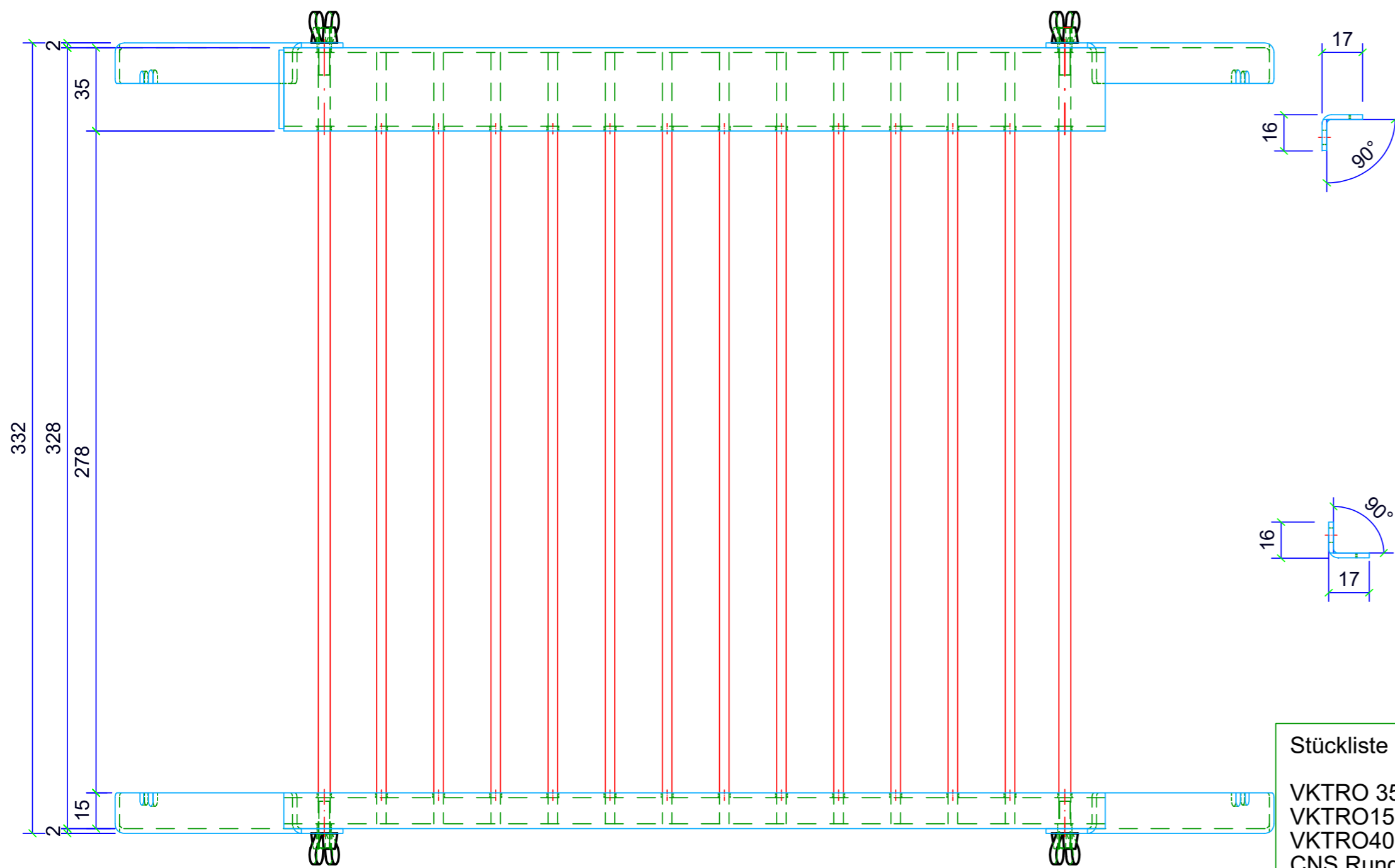
Grundriss Grill
